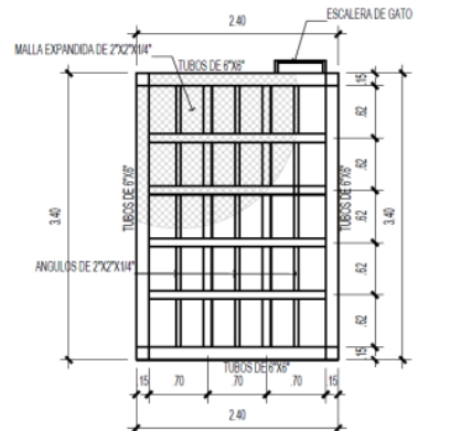
PLANTA DE ESTRUCTURA DE SOPORTE ESCALA 1:50
