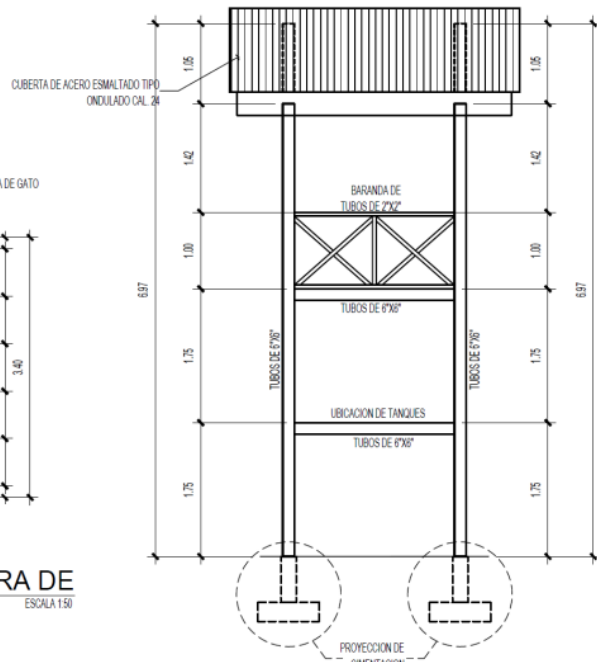
ELEVACION DE ESTRUCTURA DE SOPORTE ESCALA 1:50
