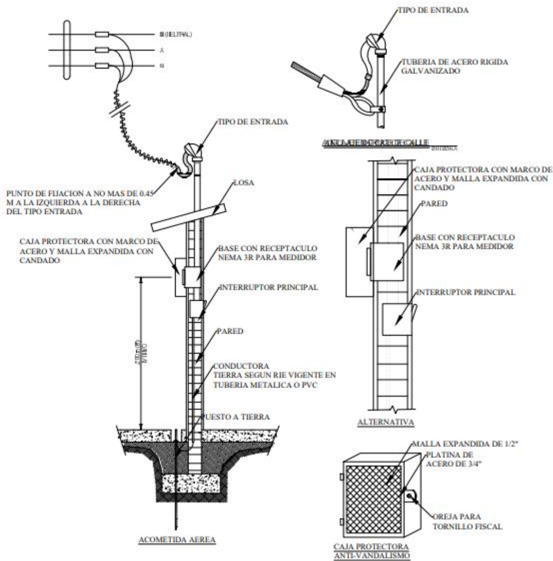
ESQUEMATICO DE LA PAREDILLA
