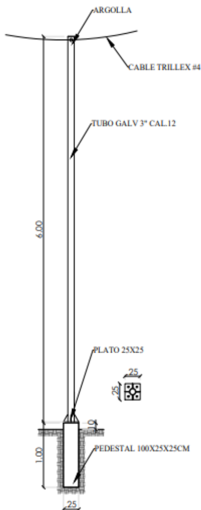
ESQUEMATICO POSTE DE LUZ
